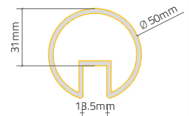
TBK GB - RC3
