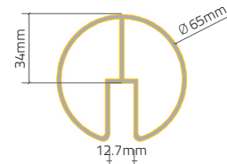
TBK GB - RC5
