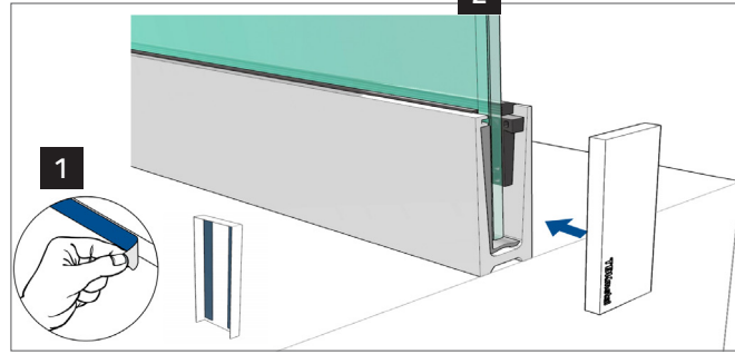
TBK GB END CAP
