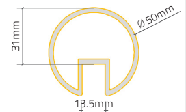
TBK GB - RC3
