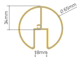
TBK GB - RC4
